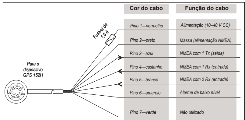
Cablagem do GPS 152H
